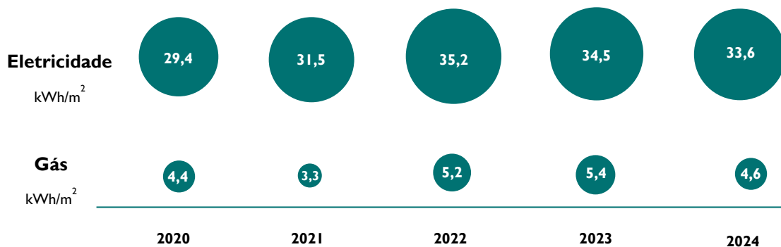
Figura 5: Consumos de energia por área utilizada
